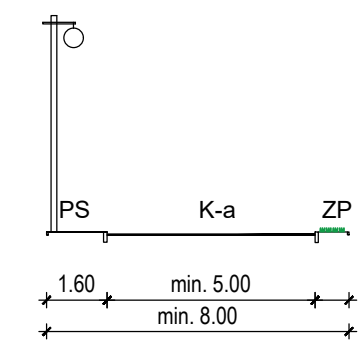
UK3 - presjek 3-3
