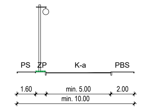
UK2 - presjek 2-2
