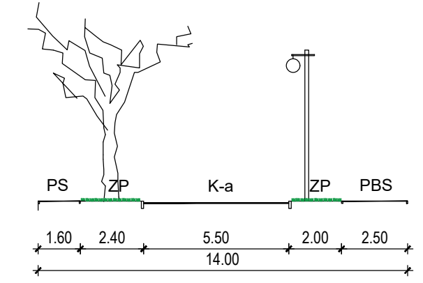
UK1 - presjek 1-1
