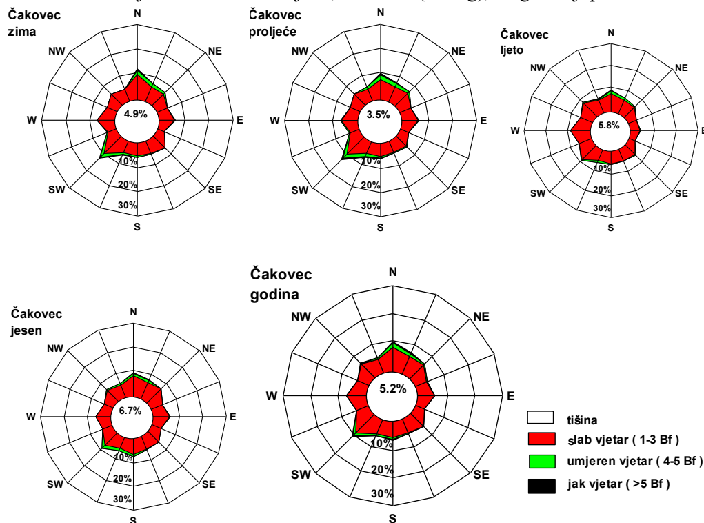
Slika 6 : Godišnja i sezonske ruže vjetera, Čakovec (Prelog), 20 godišnji period
